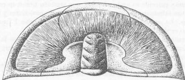
Fig. 1. — Reconstrucción del céfalo de Amecephalina argentina , en base a los ejemplares ilustrados en la lámina I, figuras 1-3. \times 3,5
