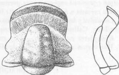
Fig. 3. — Reconstrucción del cráneos de Eteraspis prosorysa sp. nov. en base al holotipo y paratipo ilustrados en la lámina I, figuras 5-7 x 3.
