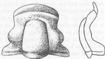
Fig. 2. — Reconstrucción del cranidio de Eteraspis orbignyana Kayser. \times 2 aproximadamente
